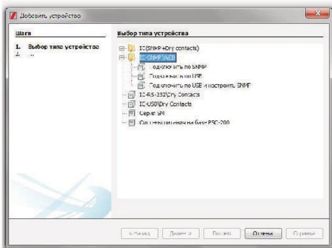
Рисунок А4б. Создание подключения устройства в ПО «Shtyl Device Manager»
